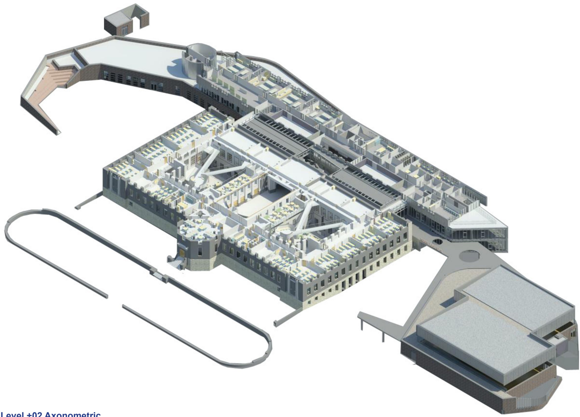
Level +02 Axonometric
